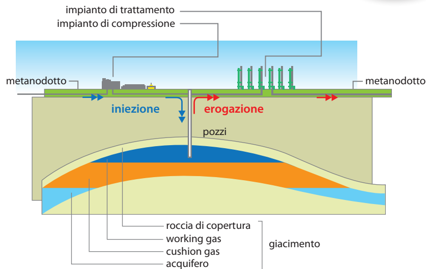
Figura 3 - Schema di un giacimento di stoccaggio (fonte Stogit)
