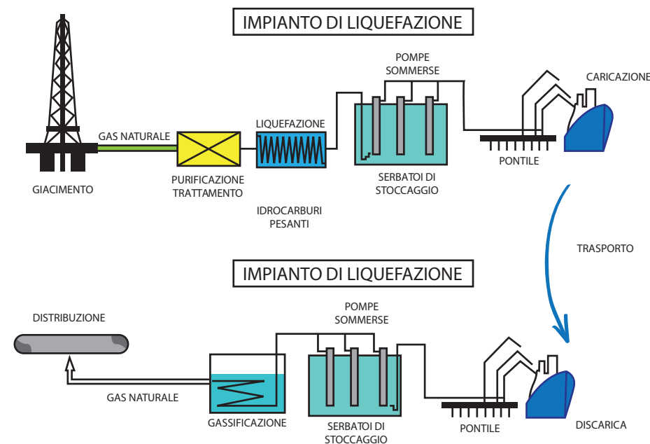
Figura 2 - Ciclo del GNL
